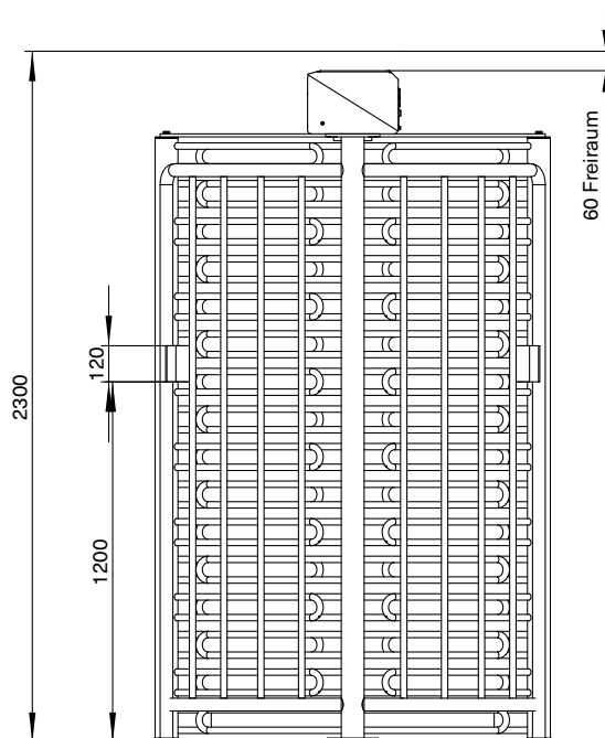
MPT 353 – versie met 3 vleugels Zijaanzicht
