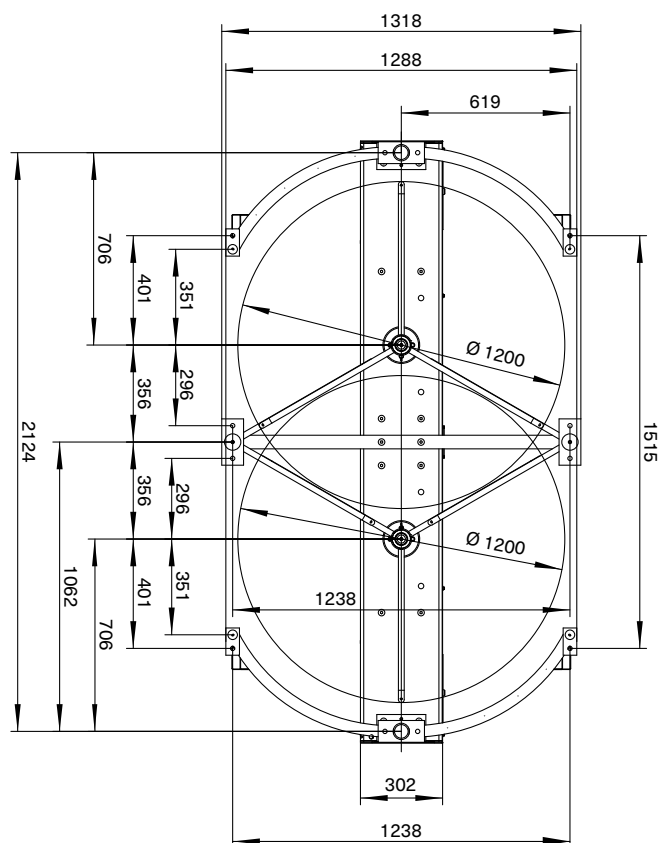
MPT 353 – versie met 3 vleugels
