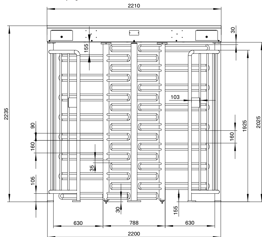
MPT 353 – versie met 3 vleugels Vooraanzicht van binnenzijde gezien
