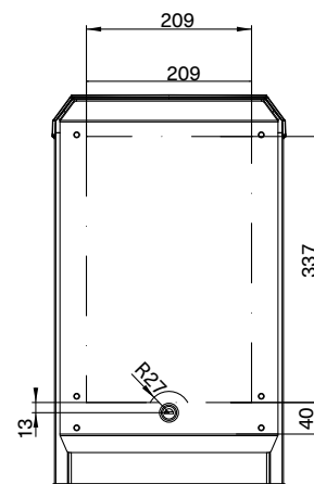
Teminal-ML: Gedetailleerd zicht van frontpaneel
