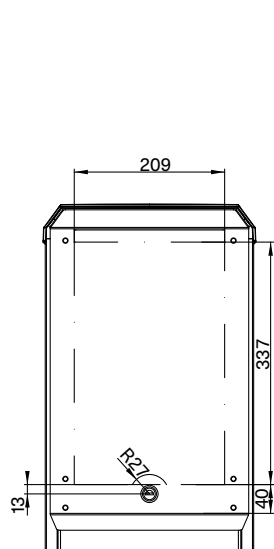
Teminal-MS: Gedetailleerd zicht van frontpaneel
