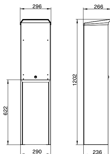
Teminal-MH: Voor- en zijaanzicht
