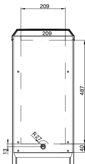
Teminal-MH: Gedetailleerd zicht van frontpaneel
