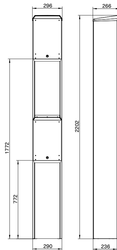
Teminal-ML: Voor- en zijaanzicht
