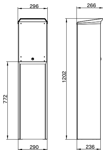
Teminal-MS: Voor- en zijaanzicht
